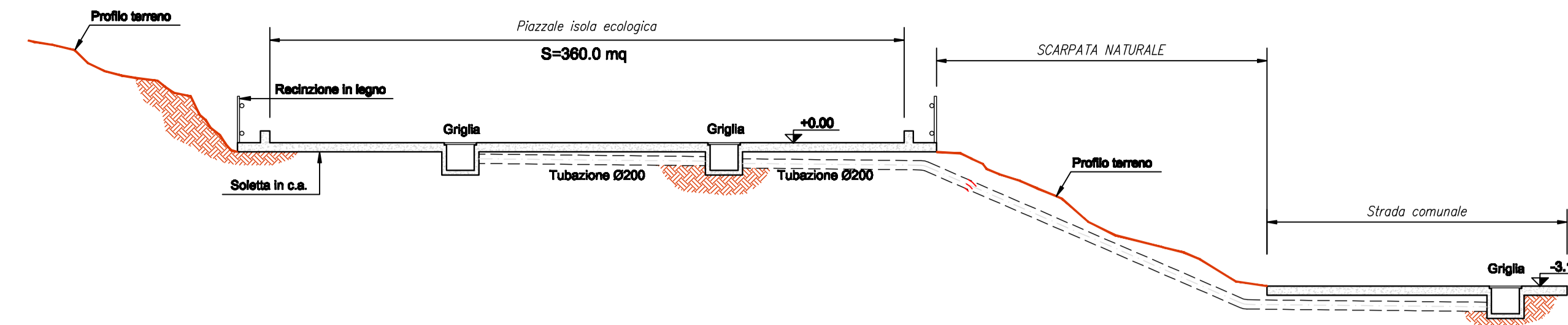
VISTA "1"
